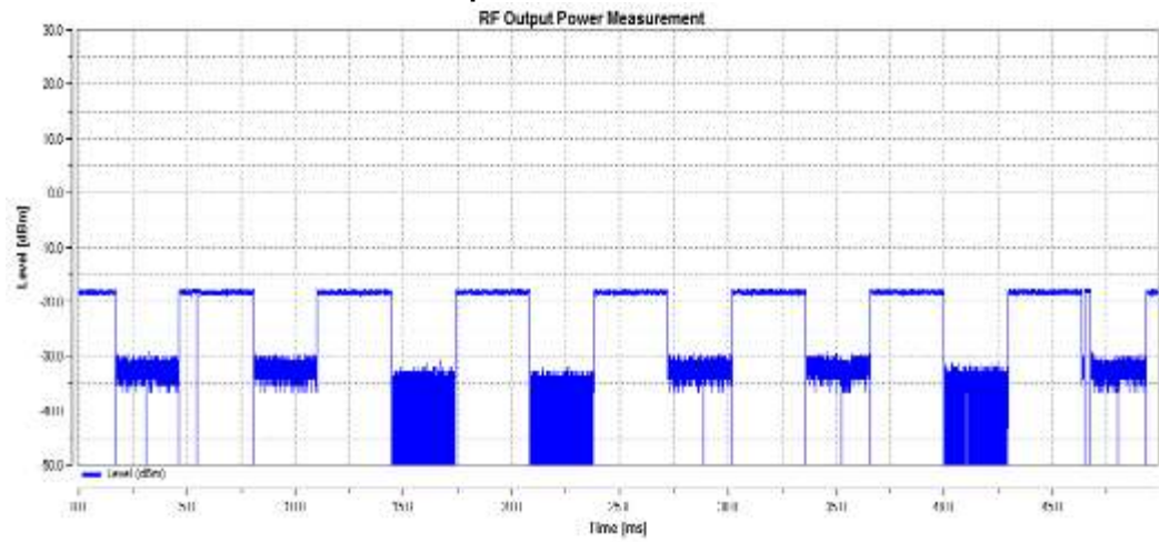
RF Output Power_TNVN_GFSK
