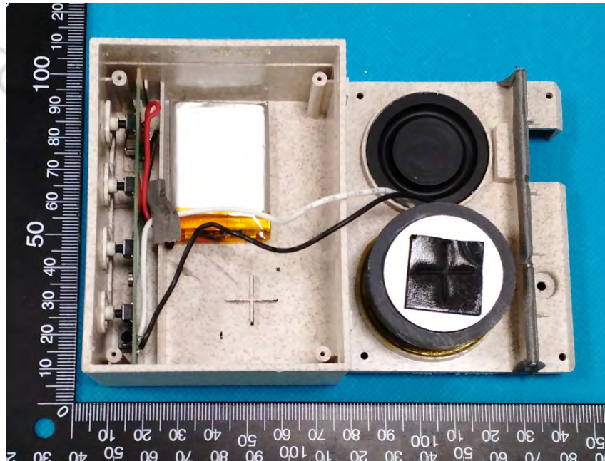
EUT Photo 6
